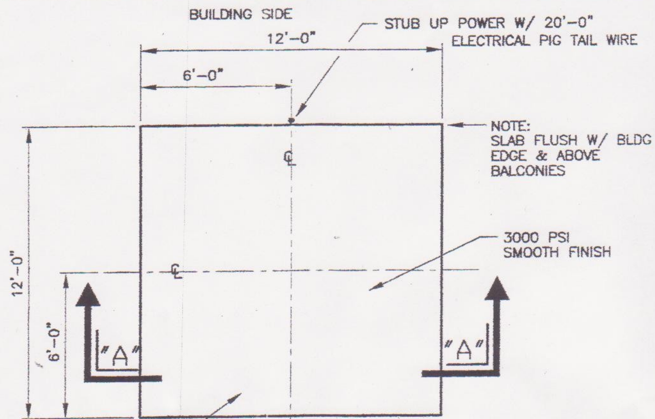
PLAN SCALE: 1/4"=1'-0"
