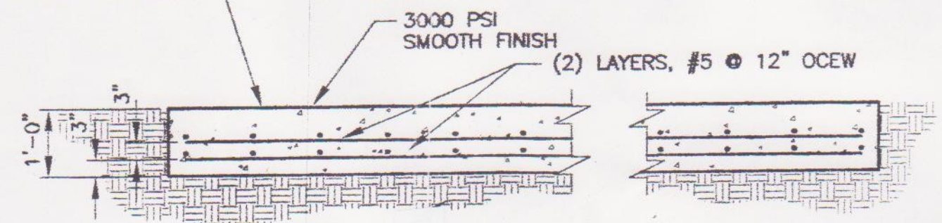
SECTION "A-A" SCALE: 1/2"=1'-0"
